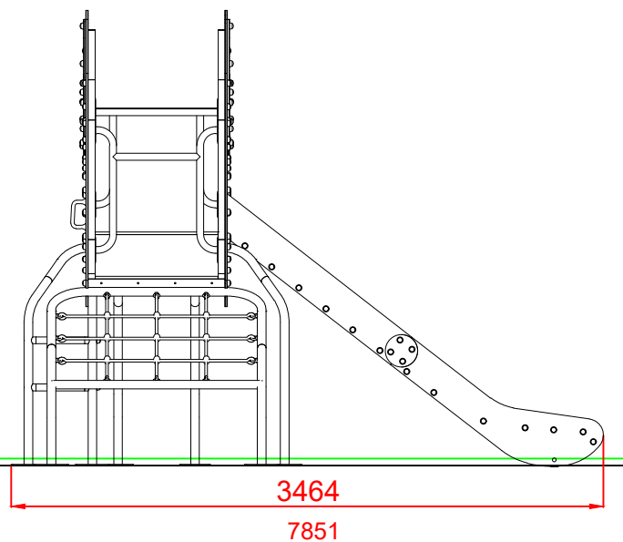
PERFIL
