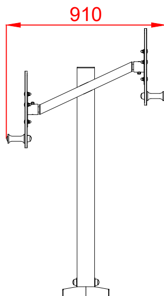
PERFIL DERECHO
