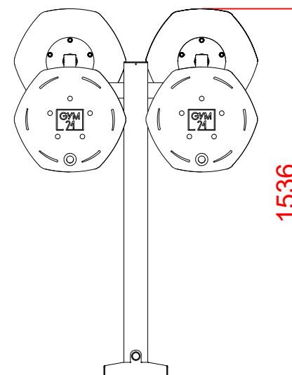
ALZADO
