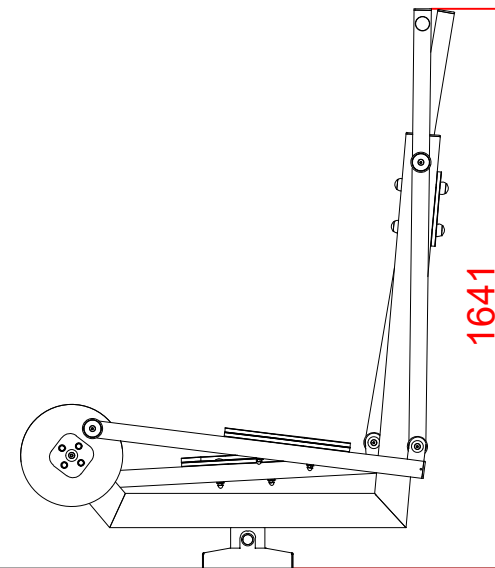
ALZADO
