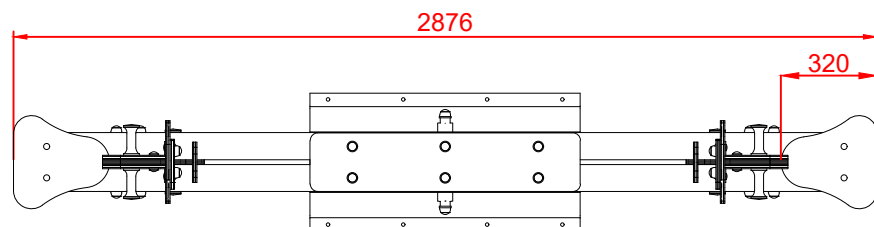
PLANTA
