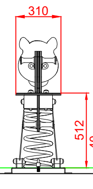
PERFIL
