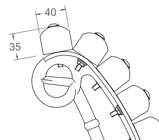
DETALLE A
