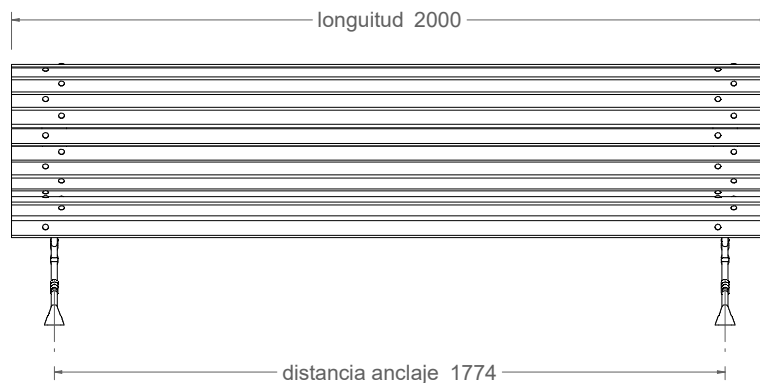
vista alzado 1:20
