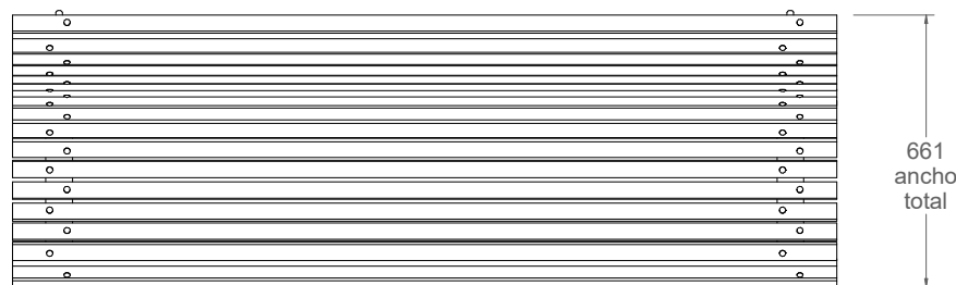
vista en planta 1:20
