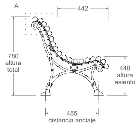
vista lateral 1:20
