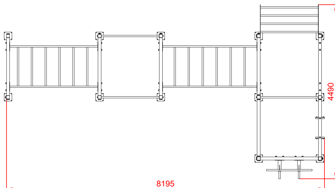
PLANTA
