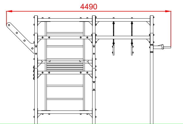
PERFIL
