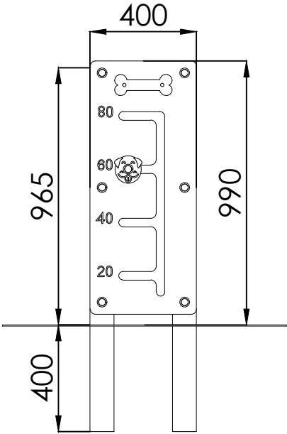
PERFIL
