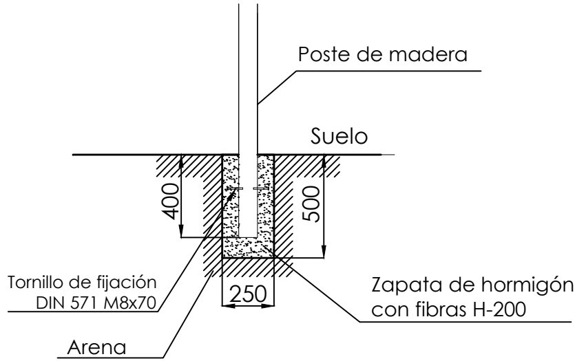
ESQUEMA DE CIMENTACIÓN
