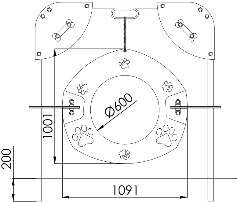
ALZADO
