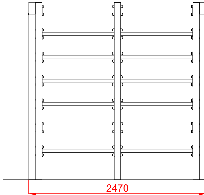
ALZADO
