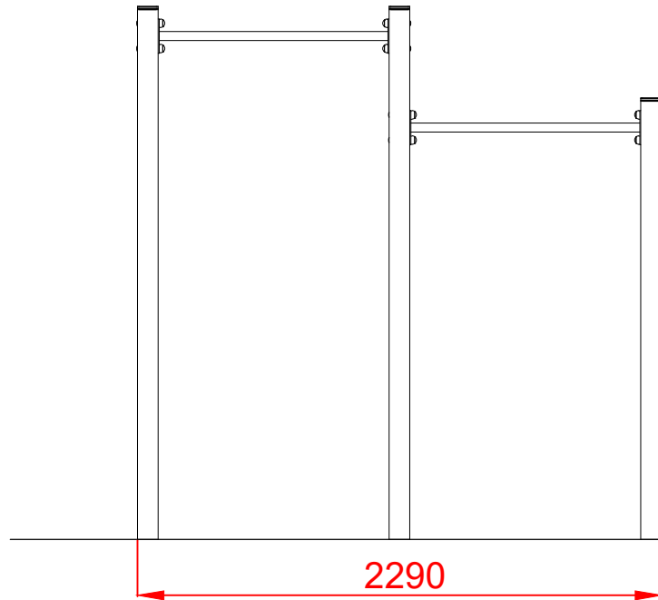
ALZADO
