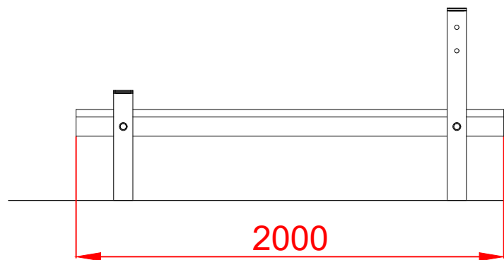
ALZADO
