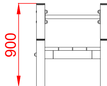
PERFIL IZQUIERDO
