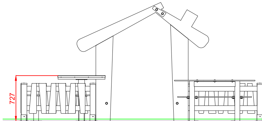
ALZADO
