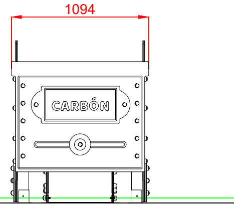
PERFIL IZQUIERDO
