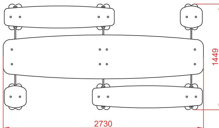
PLANTA
