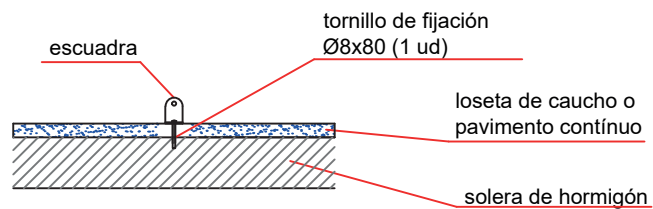
ESQUEMA DE CIMENTACIÓN EN HORMIGÓN
