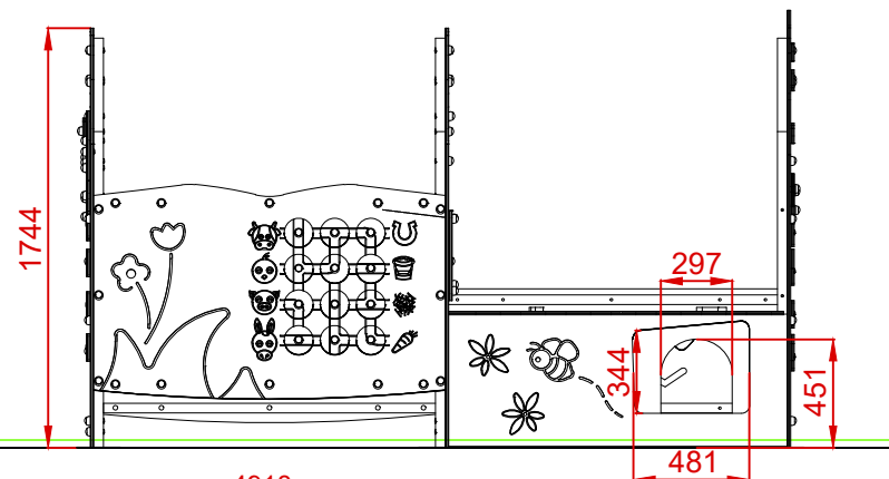
PERFIL IZQUIERDO
