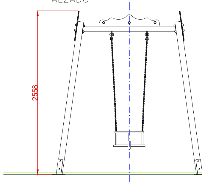
ALZADO
