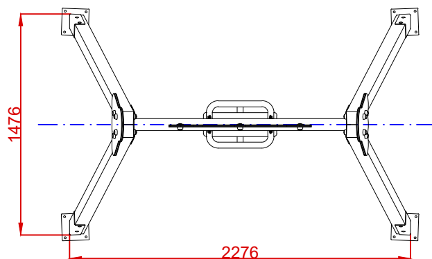
PLANTA
