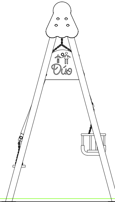
PERFIL
