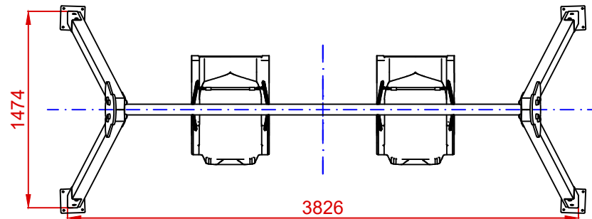
PLANTA
