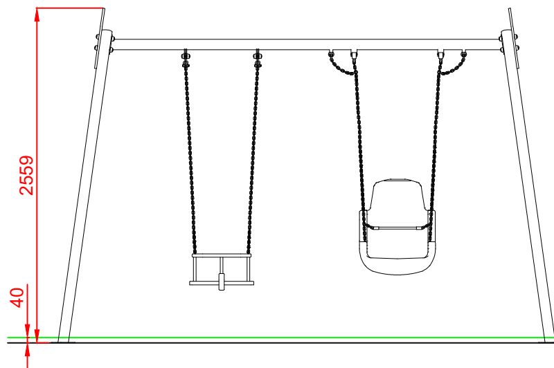
ALZADO
