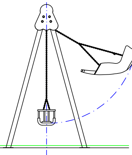
PERFIL
