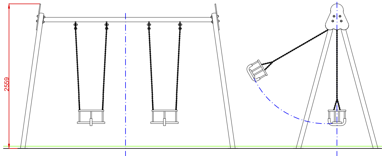
ALZADO
