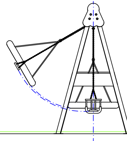
PERFIL
