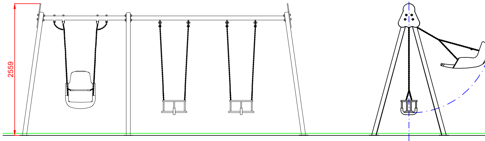
ALZADO
