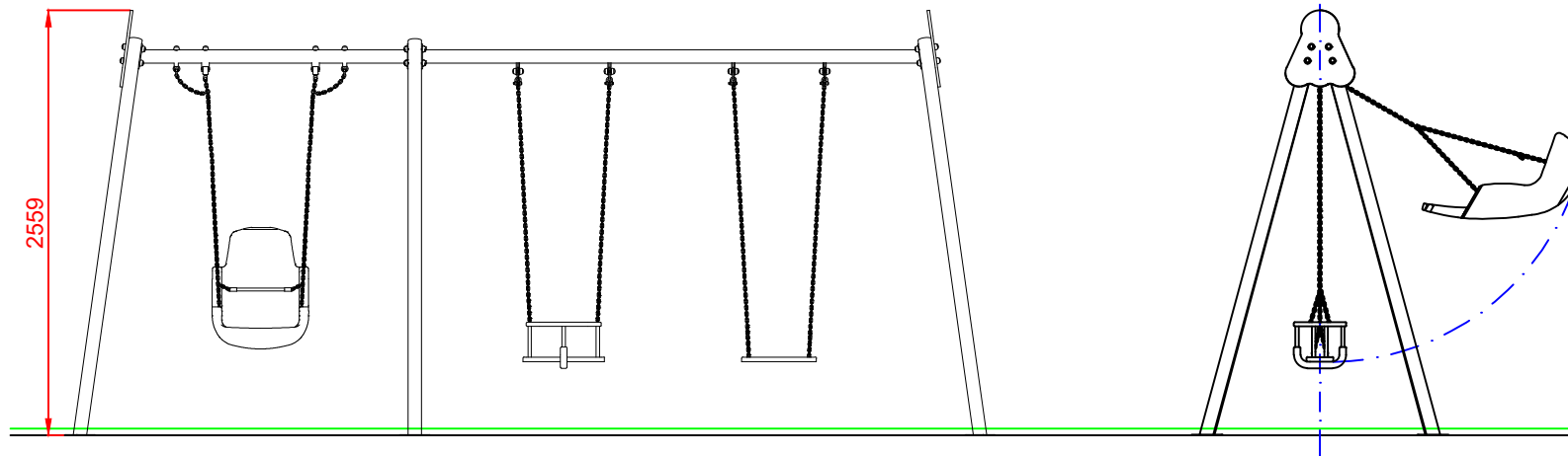
ALZADO
