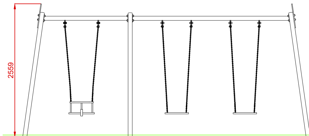
ALZADO
