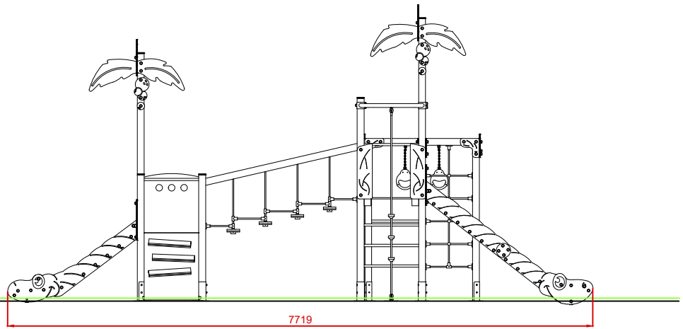
PERFIL IZQUIERDO
