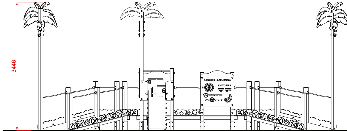
ALZADO
