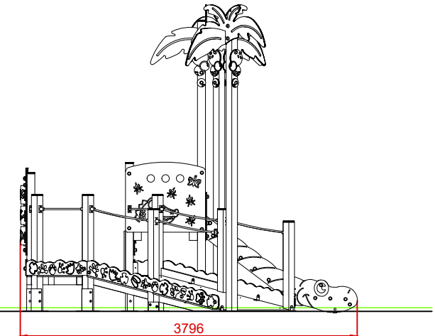
PERFIL IZQUIERDO
