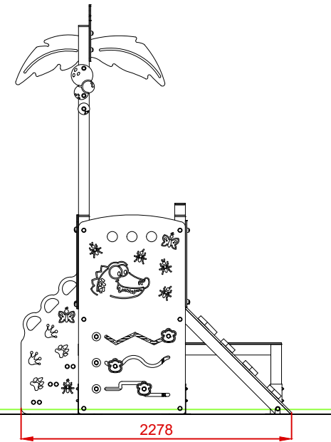
PERFIL IZQUIERDO
