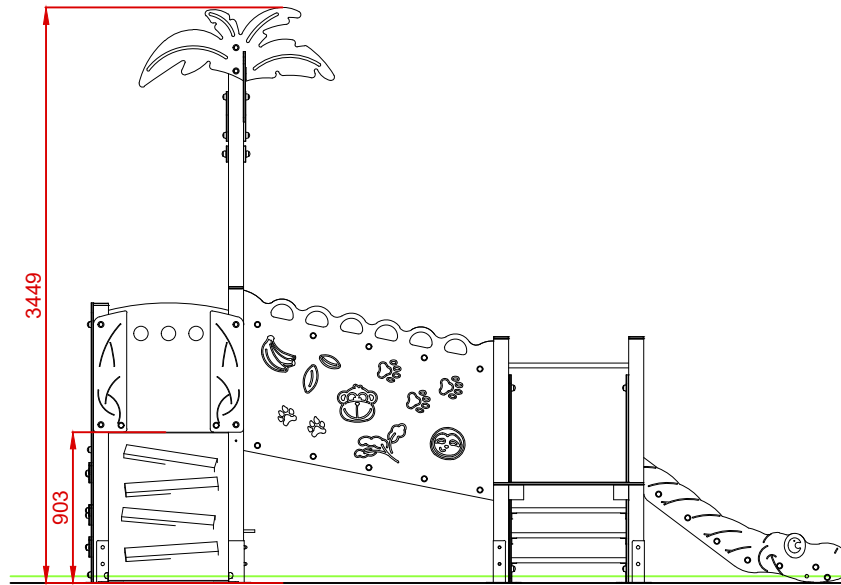
ALZADO
