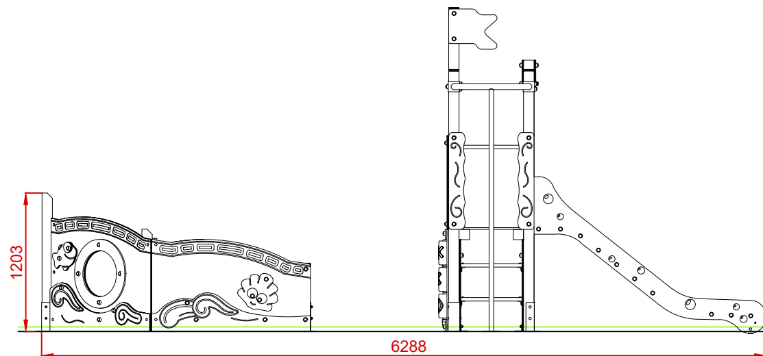
ALZADO
