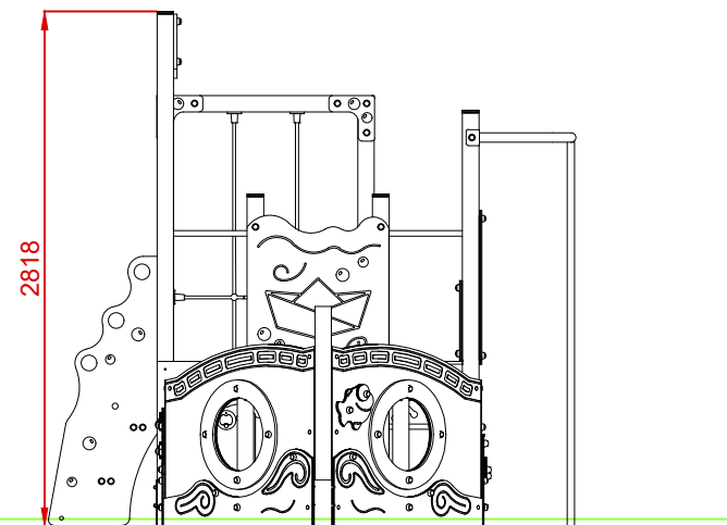
PERFIL IZQUIERDO
