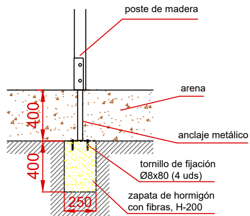
DETALLES CIMENTACIÓN ESQUEMA DE CIMENTACIÓN EN ARENA
