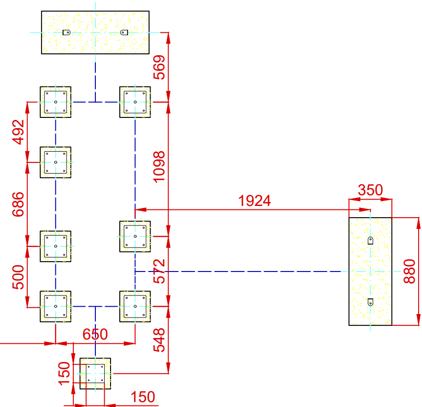
ESQUEMA DE CIMENTACIÓN EN HORMIGÓN
