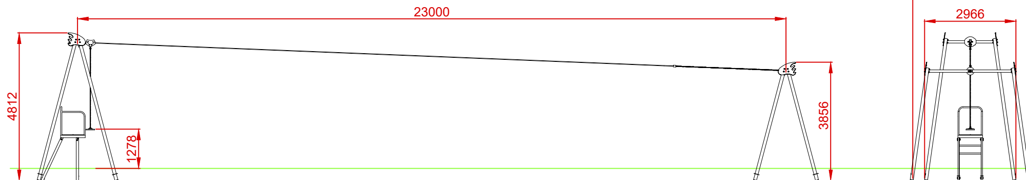
ALZADO
