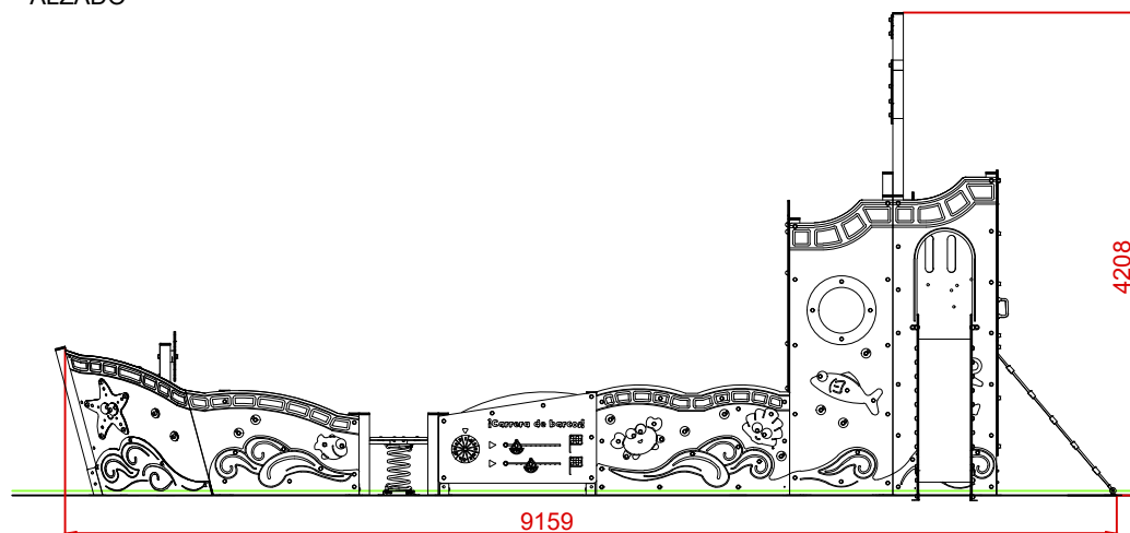
ALZADO
