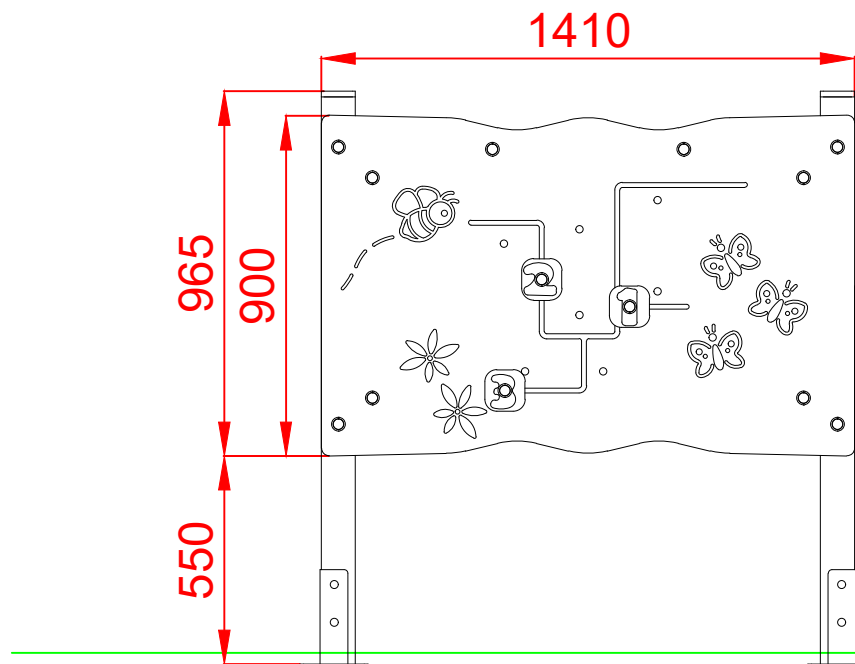
ALZADO
