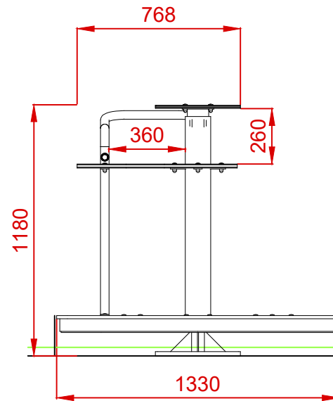
ALZADO
