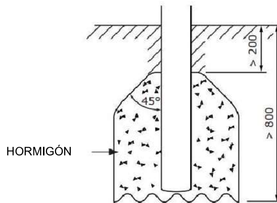
DETALLE CIMENTACIÓN
