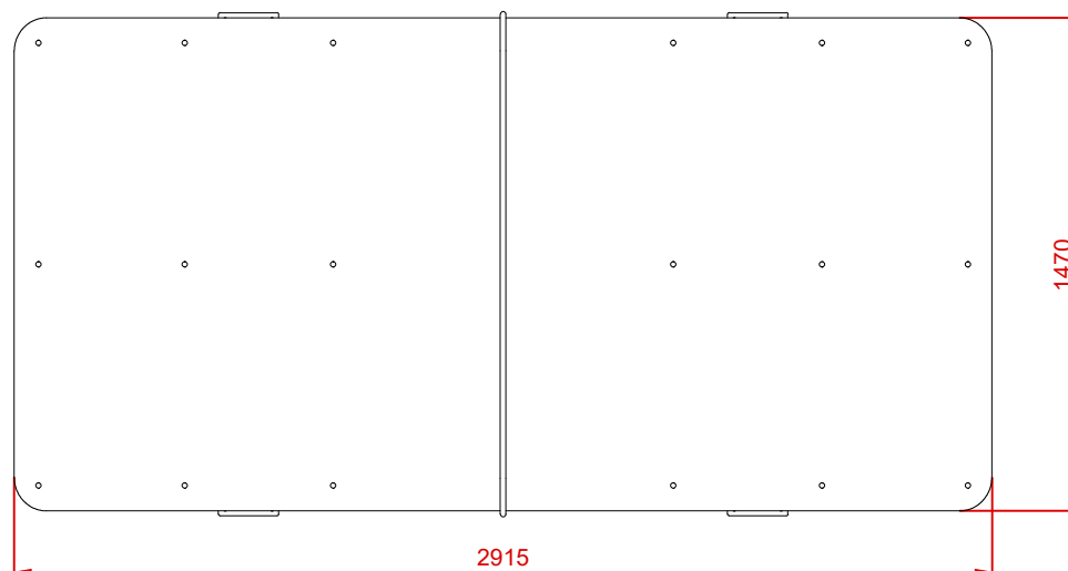
PLANTA
