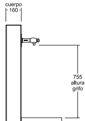
vista lateral 1:20
