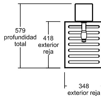
vista en planta 1:20
