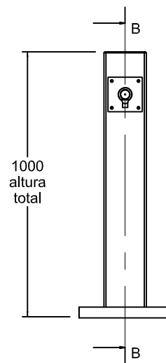
vista alzado 1:20
