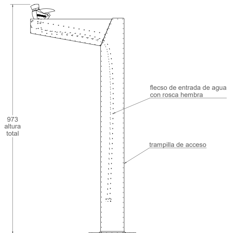
vista lateral 1:10
