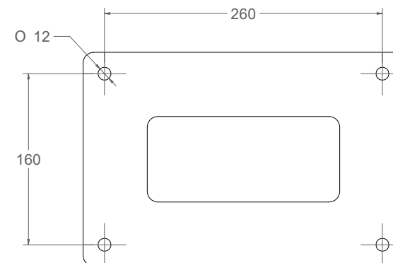
detalle anclaje 1:5
