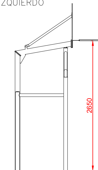
PERFIL IZQUIERDO
