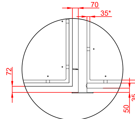
DETALLE A 1:2
