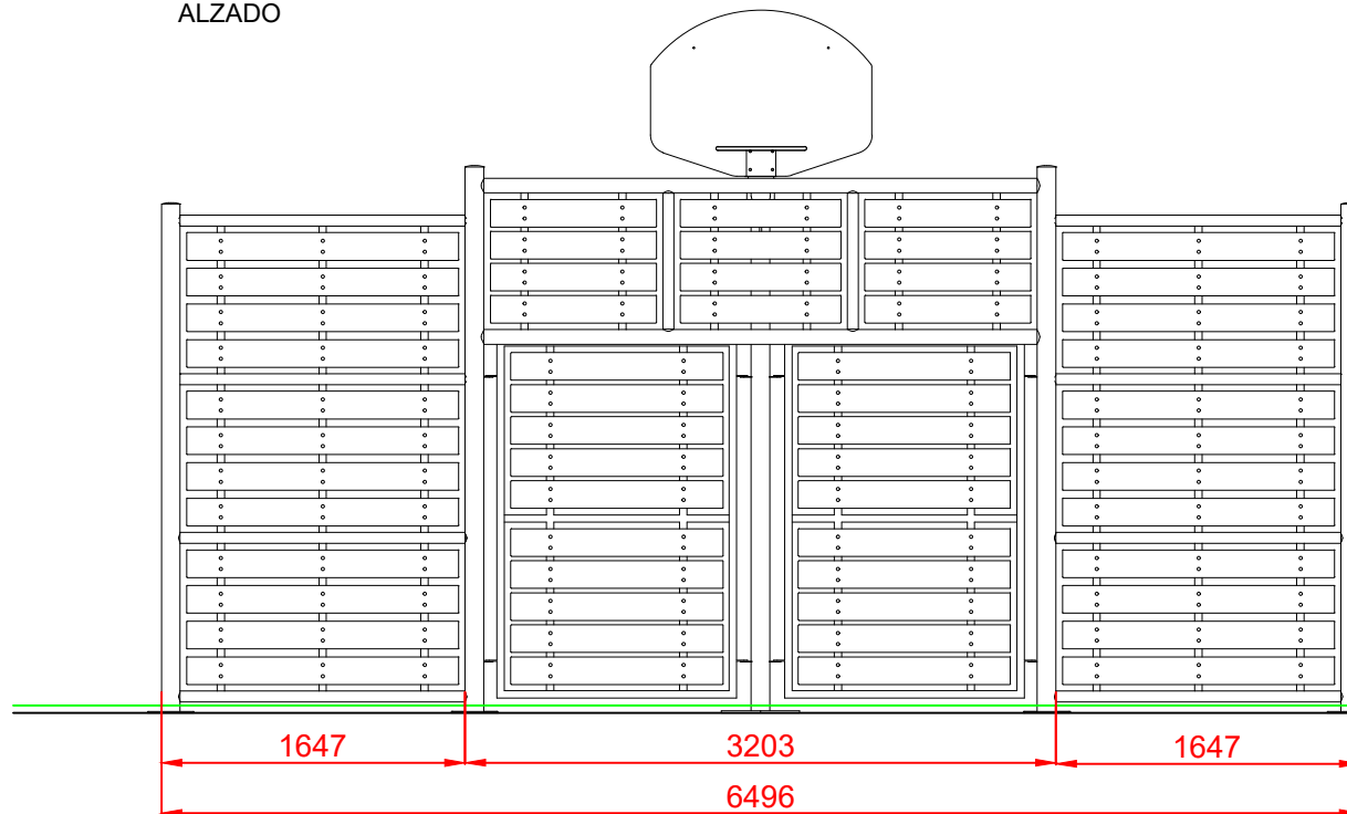
ALZADO
