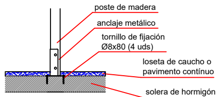
ESQUEMA DE CIMENTACIÓN EN HORMIGÓN
