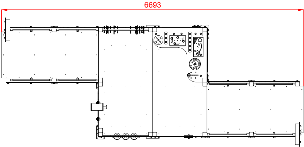
PLANTA
