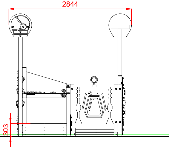
PERFIL IZQUIERDO
