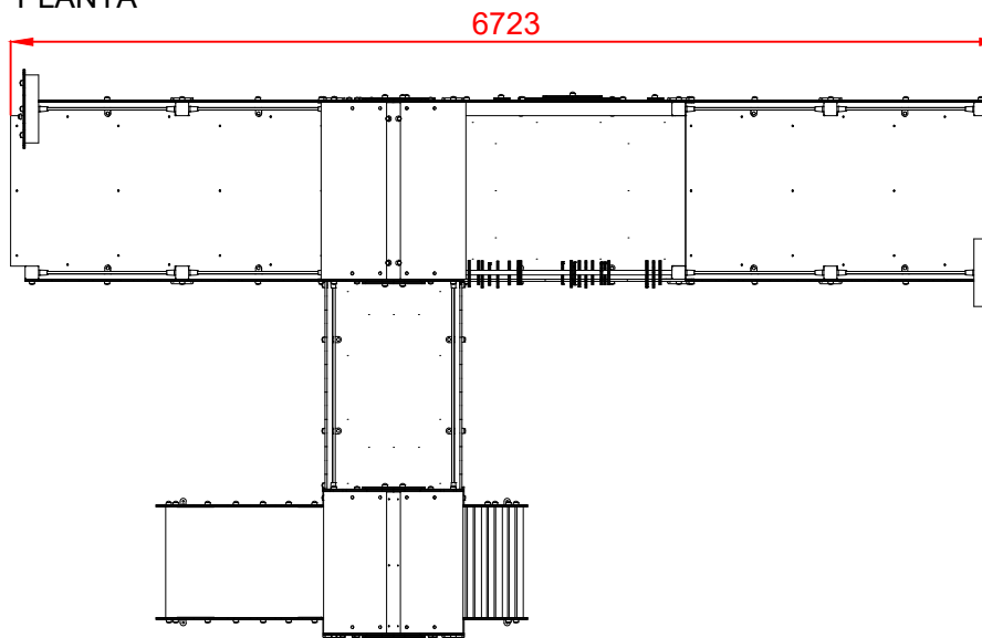
PLANTA
