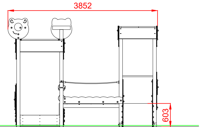
PERFIL IZQUIERDO
