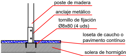
ESQUEMA DE CIMENTACIÓN EN HORMIGÓN
