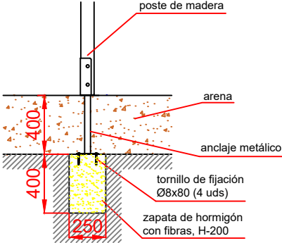
ESQUEMA DE CIMENTACIÓN EN ARENA
