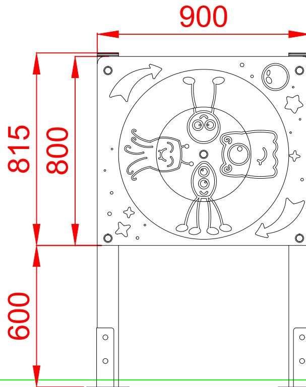
ALZADO
