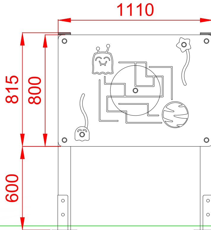
ALZADO
