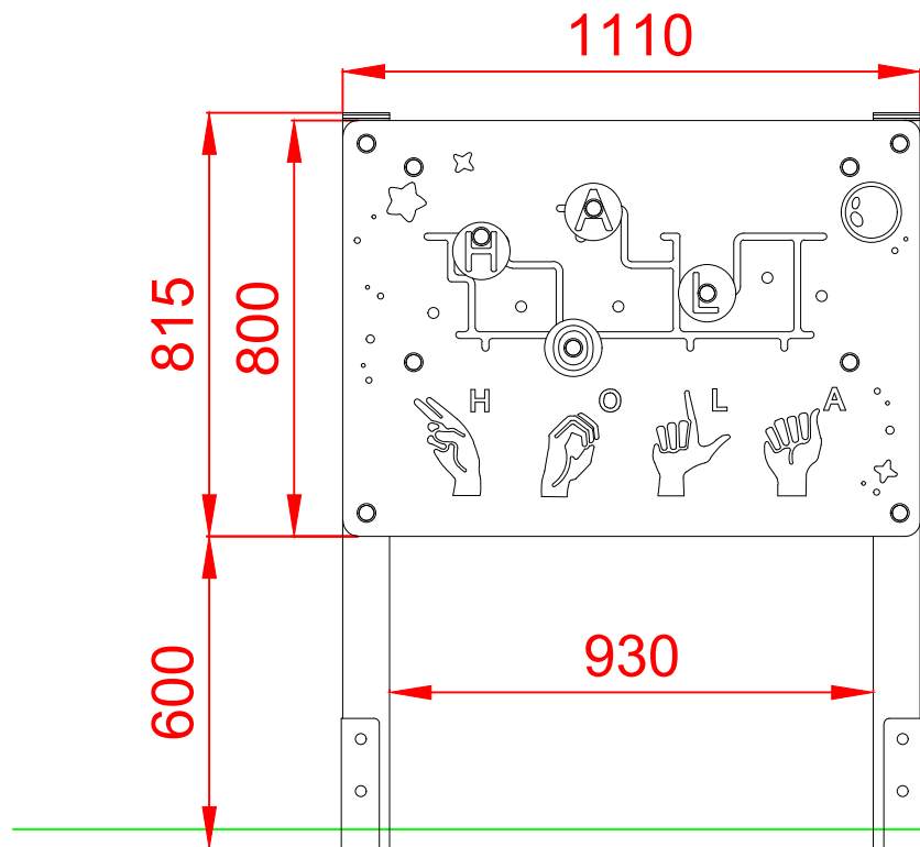
ALZADO
