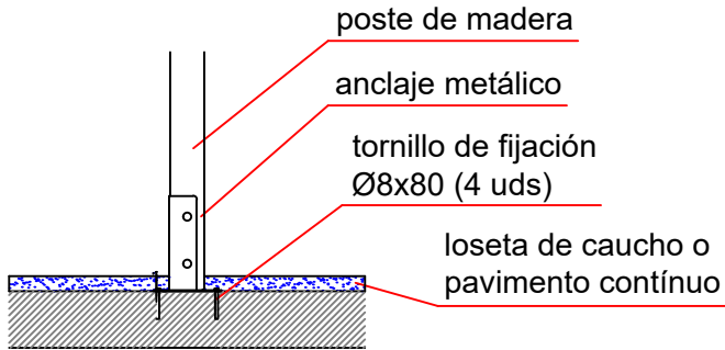
ESQUEMA DE CIMENTACIÓN EN HORMIGÓN
