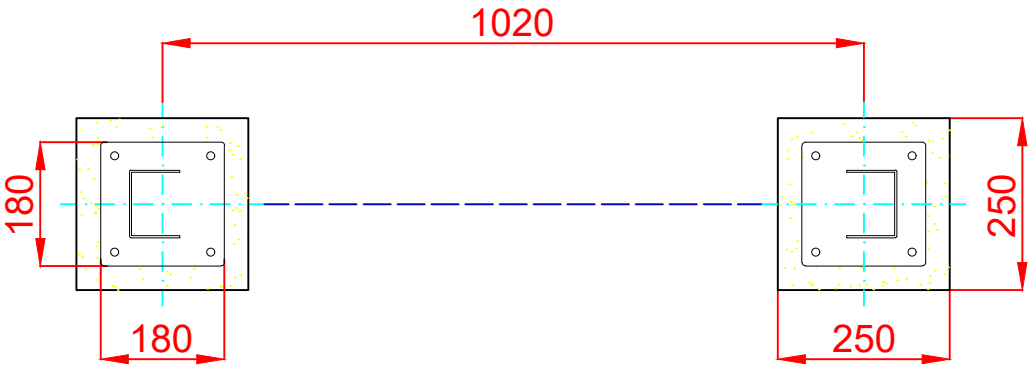
PLANTA CIMENTACIÓN
