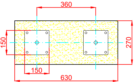
PLANTA DE CIMENTACIÓN E: 2/1
