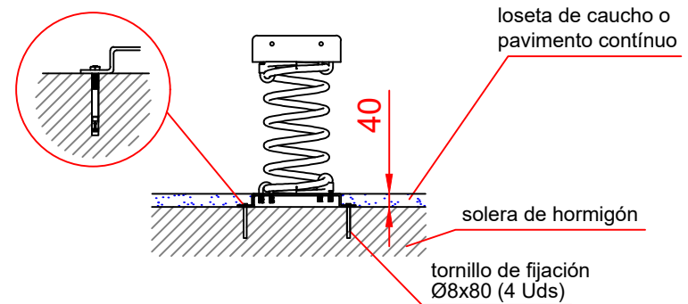
Detalle de sujeción de espiral metálico
