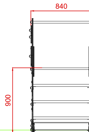
PERFIL
