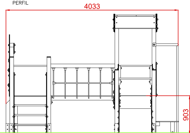
PERFIL
