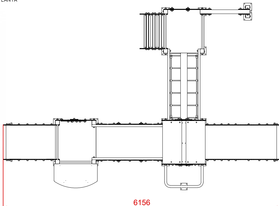
PLANTA
